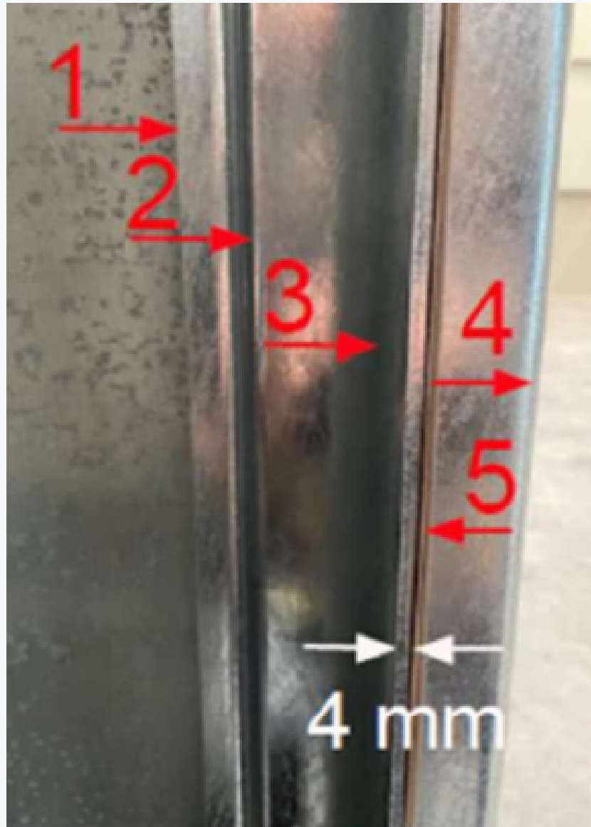
Hoekprofielen, uit één stuk met 5 zettingen
